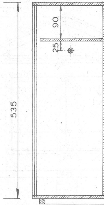
DOORSNEDE
